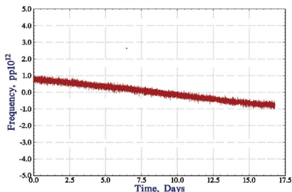
上图为16天连续运行的频率偏差曲线
