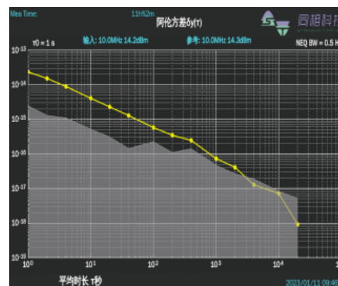
稳定度本底(典型值)
